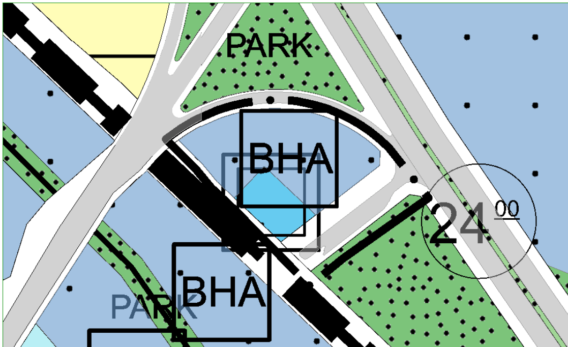
Şekil 3 Öneri 1/5000 Ölçekli Nazım İmar Planı değişikliği
